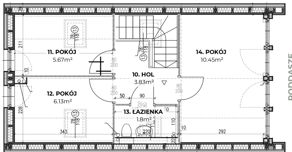
RZUTY
