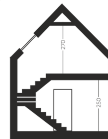
PRZEKRÓJ
